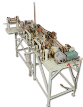
京都大学化学研究所「ビニロン」関係資料 [ca.1942-1943].より 標題: ビニロン紡糸実験装置 資料番号: ICR MIXED 2014/8/2
